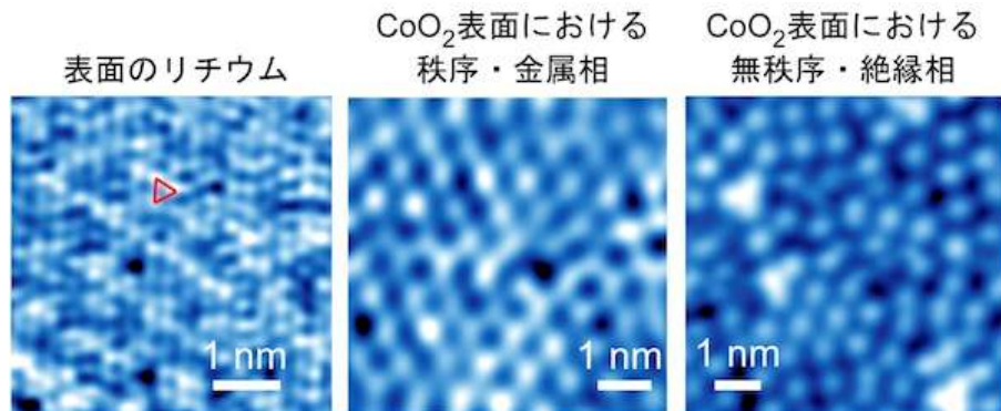
図2 コバルト酸リチウムの原子像。(左) 表面のリチウム。三角格子を組んでいる。赤の三角は図1右の三角と同じ位置を示す。(中) \text{CoO}_2 面における金属的な領域。電子秩序が形成されている。(右) \text{CoO}_2 面における絶縁的な領域。電子は無秩序に配列している。
